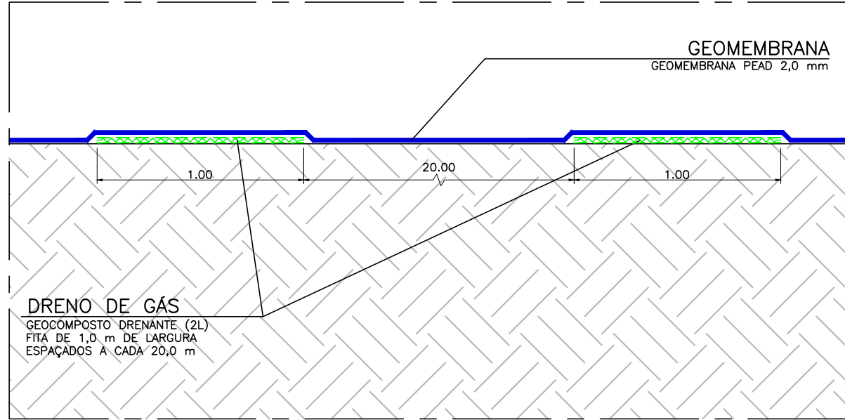
DETALHE 3 – DRENO GÁS ESCALA 1:25
