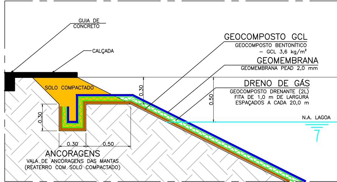
DETALHE 1 – ANCORAGEM DA GEOMEMBRANA NA CRISTA DO TALUDE ESCALA 1:25
