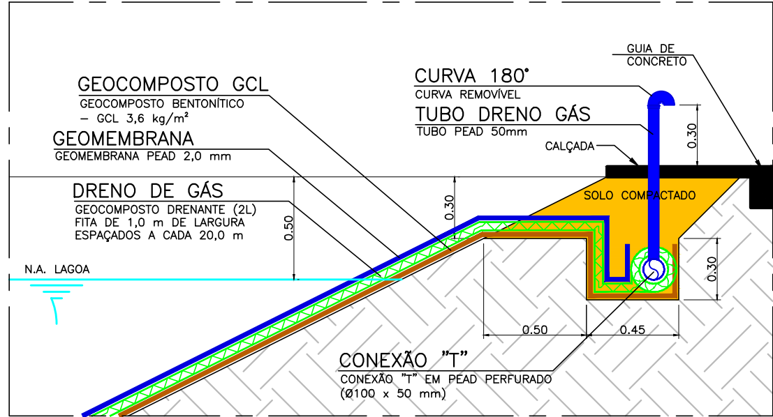
DETALHE 4 – SAÍDA DRENO DE GÁS ESCALA 1:25
