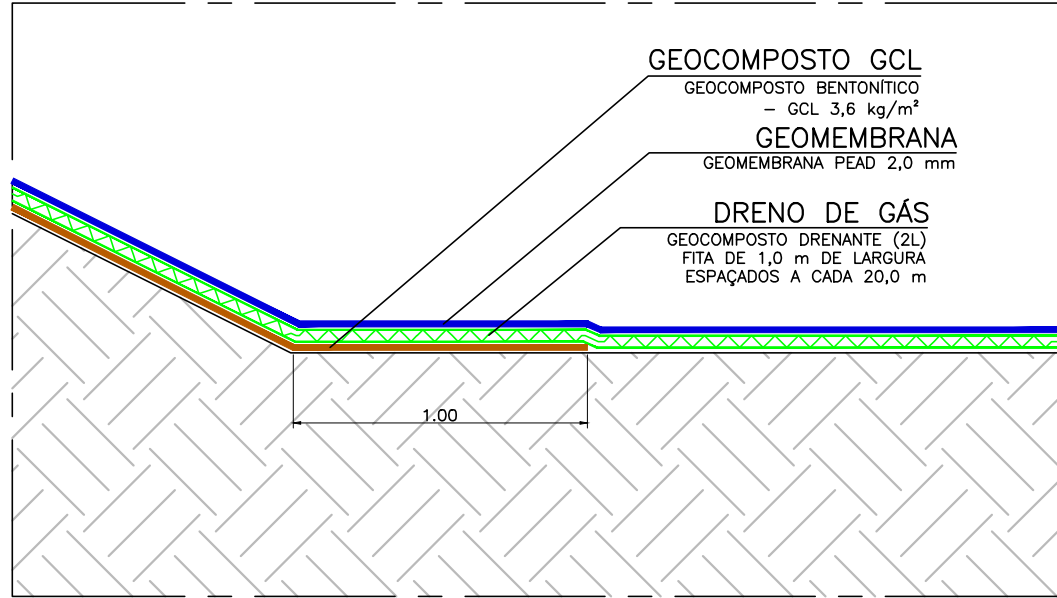
DETALHE 2 – PÉ DO TALUDE E FUNDO ESCALA 1:25
