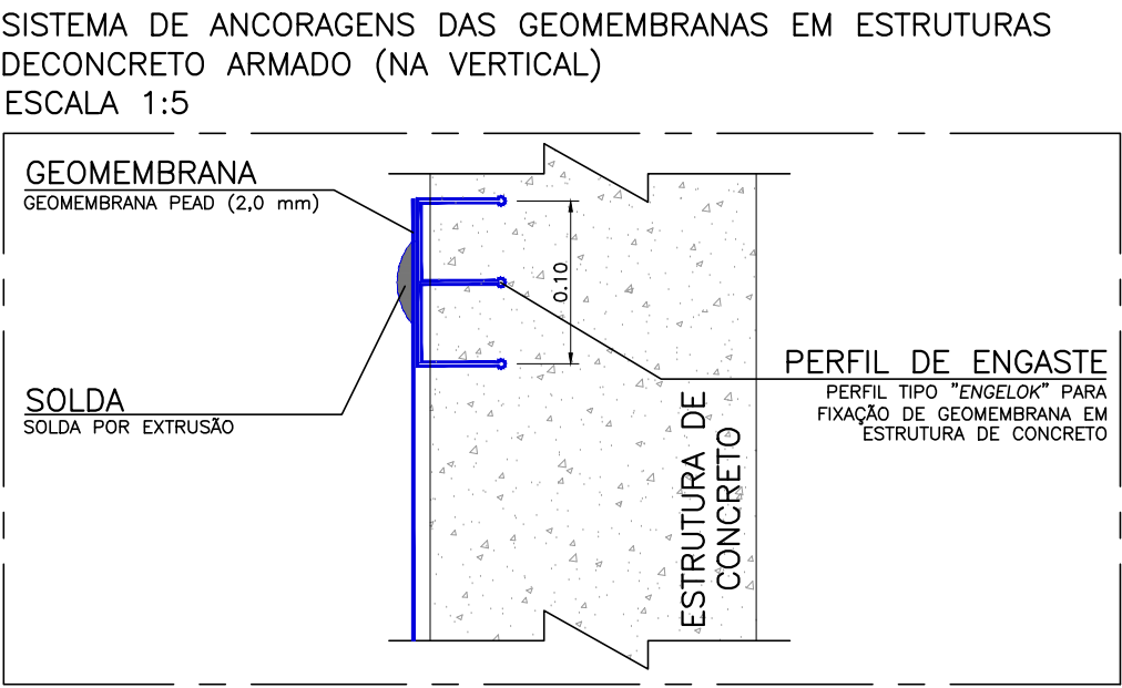
DETALHES 5 – ENGASTE DA GEOMEMBRANA
