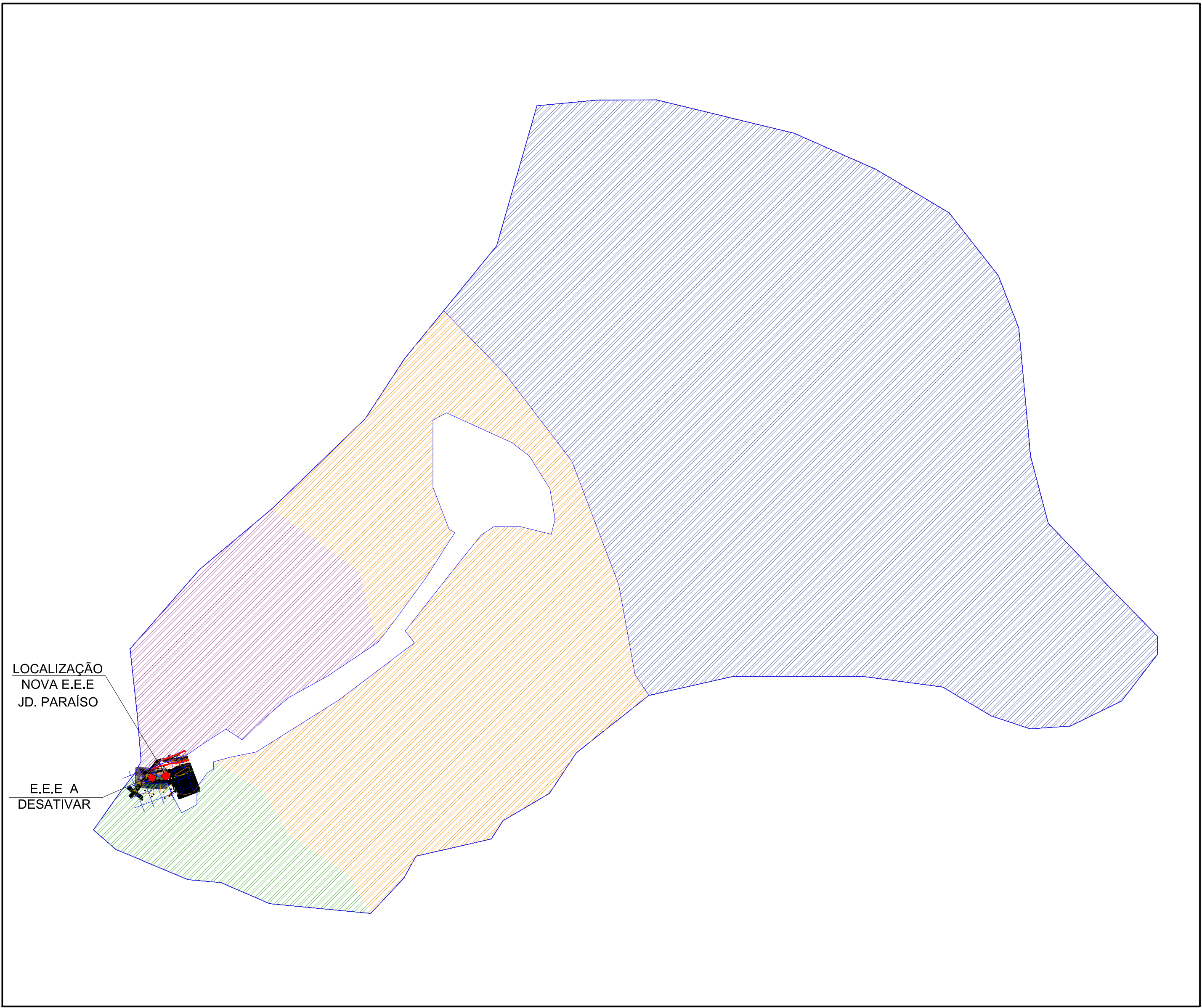
PLANTA GERAL DA BACIA DE CONTRIBUIÇÃO PARA A EEB JARDIM PARAÍSO – SOBRE CARTA DE LEVANTAMENTO AEROFOTOGRAFÉTRICO DO IGC–SP ESCALA 1:15.000
