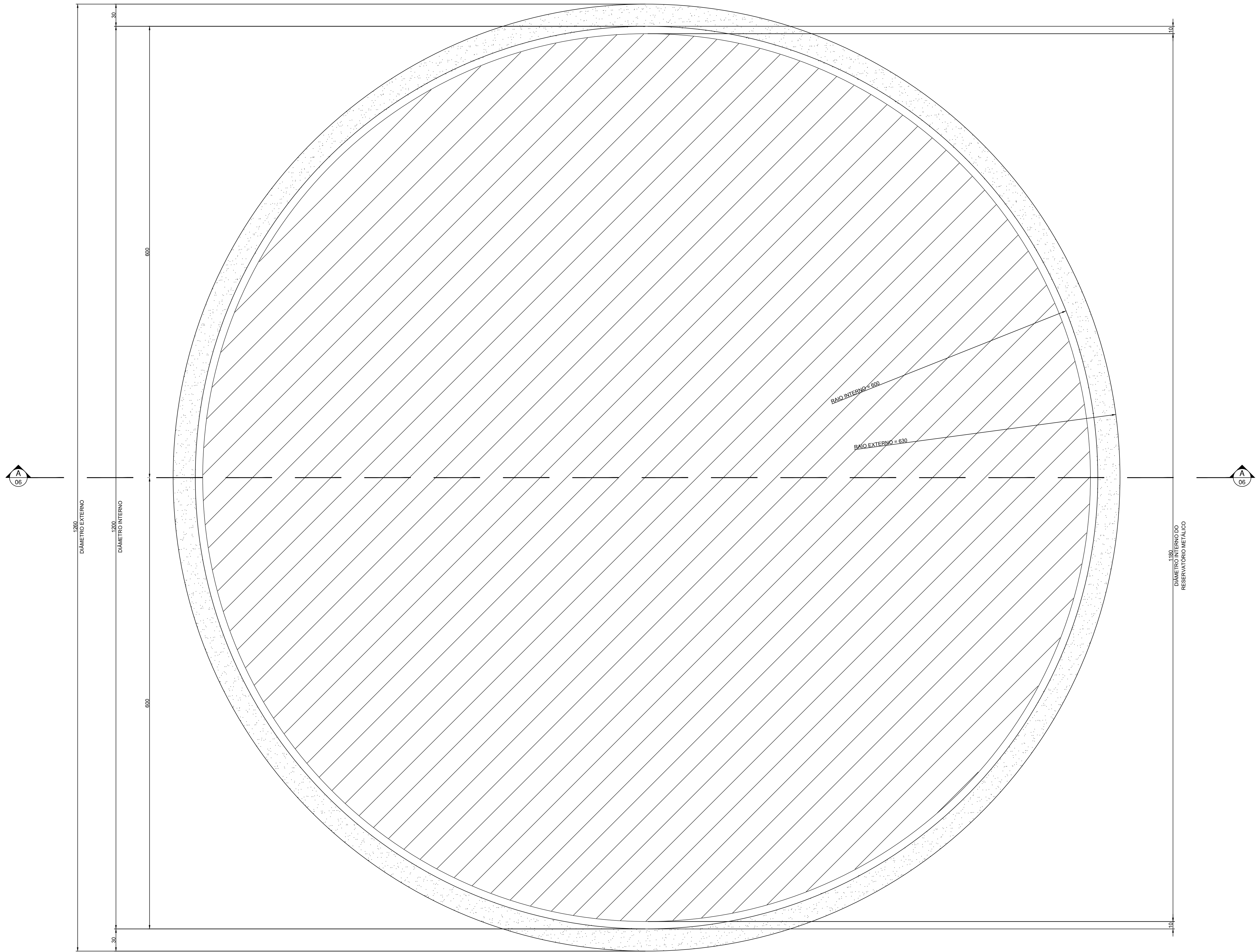
PLANTA - BASE DO RESERVATÓRIO 1.000m² ESCALA 1:25
