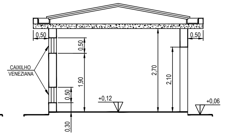
CORTE B-B
