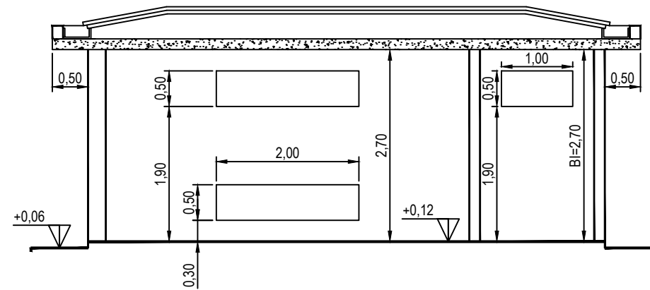
CORTE A-A
